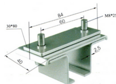
Carro de Arrastre Código C32106
