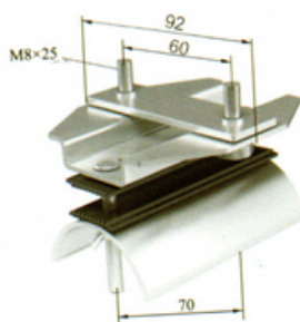
Portacable de Inicio Condigo C40104
