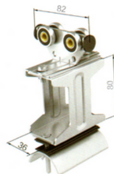
Carro de Arrastre Código C32106
