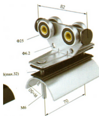
Carro Portacable Plano Codigo C32105
