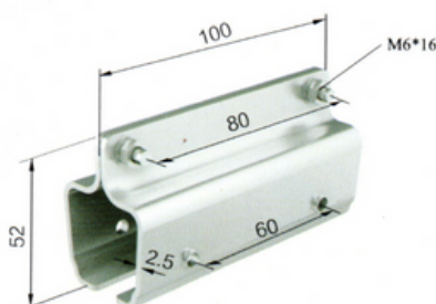
Unión para Riel C32 Código C32102
