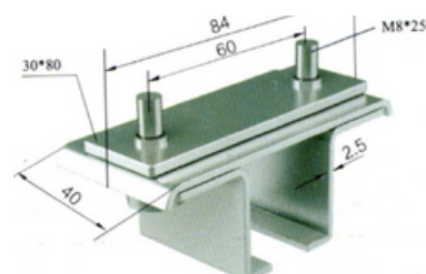
Carro de Arrastre Código C40106
