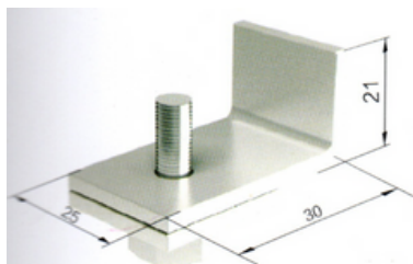
Carro Portacable Plano Codigo C40105
