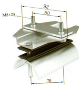
Portacable de Inicio Condigo C32104
