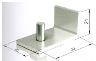
Carro Portacable Plano Codigo C32105
