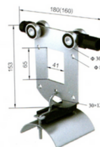
Carro de Arrastre Código C40106
